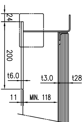
SECTION D-D 1:5
